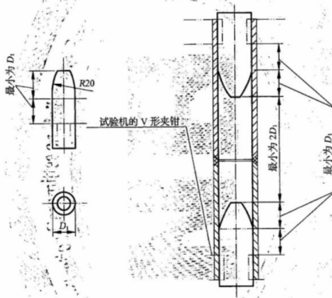
图6 管接头全截面拉伸试样
