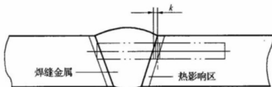
图 12 热影响区冲击试样缺口轴线位置
