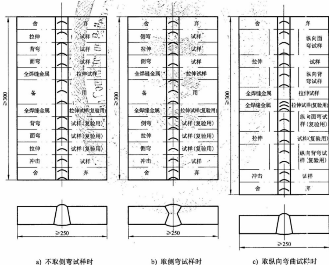
图 1 板状试件尺寸和试样位置图
